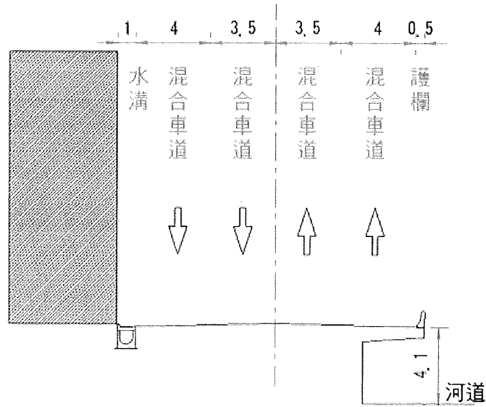
圖 1 現況道路標準斷面圖
