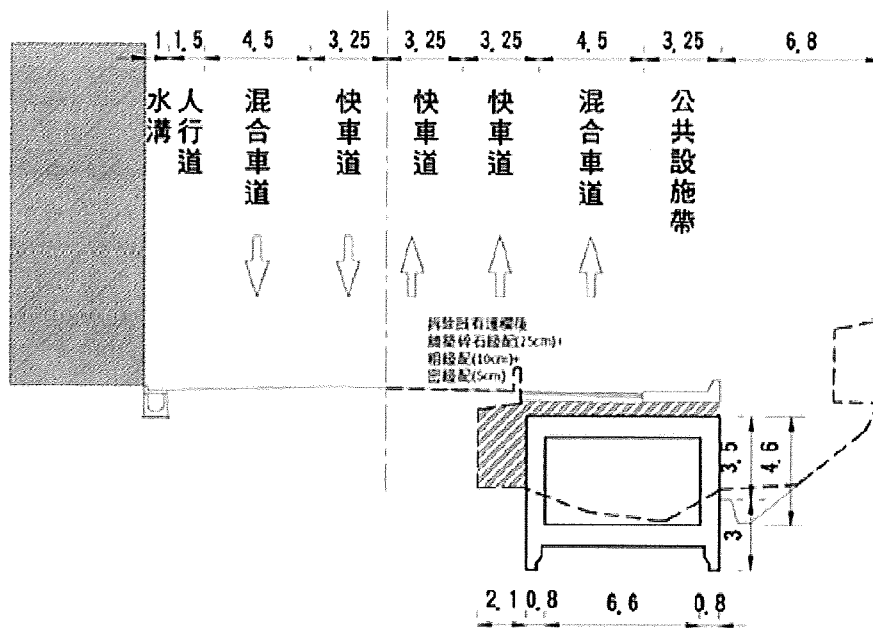
圖 2 本計畫完工後道路配置斷面圖
